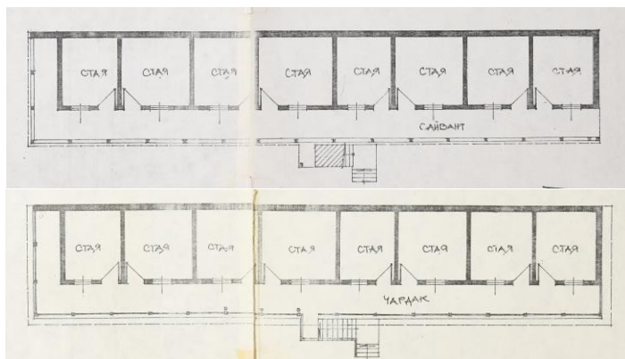
Фиг. 27 Хан – разпределение на първо и второ ниво. Извадка от досие на НКЦ, „Къща на наследниците на Марин Нанов (Хан)“, ПД-607-6-I, деклариран с писмо от 1987 г.
