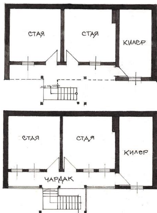
Фиг. 22 Двуетажна жилищно-стопанска сграда – план приземие и първи етаж. Извадка от досието на „Къща на Иван Недков Мичев“, ПД-0-13-II, свалена от списъка на НКЦ през 1987 г.
