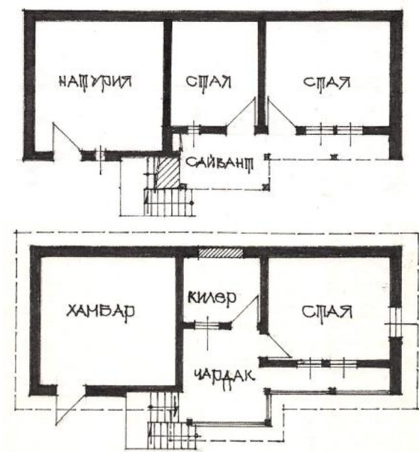
Фиг. 23 Двуетажна жилищно-стопанска сграда – план приземие и първи етаж. Извадка от досието на „Къща на Марко Петров Колев“, ПД-604-3-I, декларирана със списък през 1987 г.
